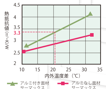
日射面の熱抵抗値比較 (厚さ 50 mm)
